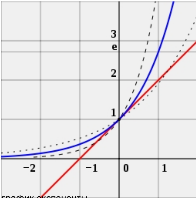
График экспоненты
